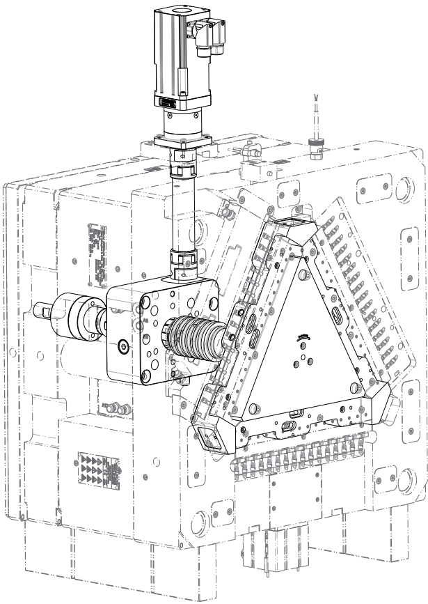
Konrad Häupler GmbH & Co. KG, Nürnberg indexing plate – 120° rotation
