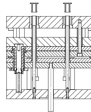
SECTION D-D
